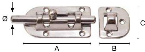
FECHO DE CULATRA INOX AISI316 MS0818
