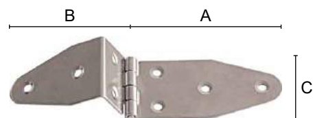
DOBRADIÇA INOX COM RESALTO AISI316 25541
