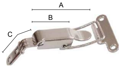
FECHO BAÚ INOX AISI304 S1300
