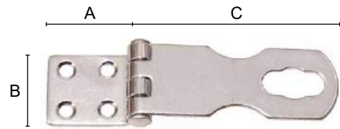
DOBRADIÇA INOX PARA CADEADO AISI316 MS0813
